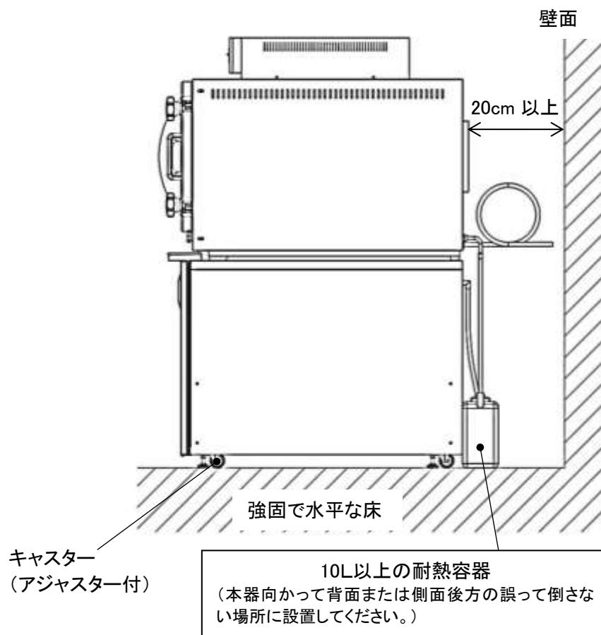
図 2 耐熱容器を使う場合の設置例
